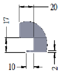
細部放大圖I 比例 1:2
